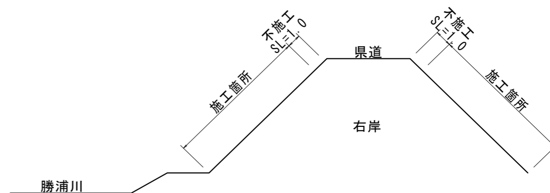
標準断面図(参考)
